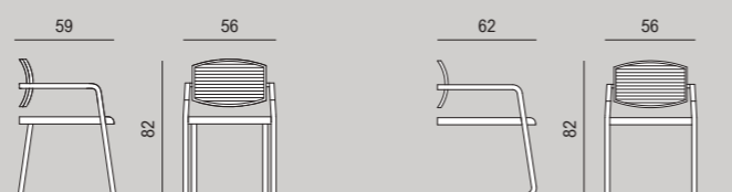
SEDUTA ATTESA + SEDUTA VISITATORE CANTILEVER IN RETE | VISITOR CHAIR, MESH BACKREST 4 LEGS + SKID FRAME
