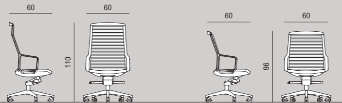
SEDUTA DIREZIONALE E SEMIDIREZIONALE IN RETE | EXECUTIVE AND MANAGER ARMCHAIR, MESH BACKREST
