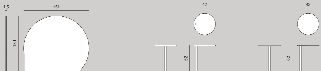
PARAVENTO + TAVOLINO CON E SENZA CARICATORE | WINDSCREEN + WAITING TABLE WITH AND WITHOUT CHARGER
