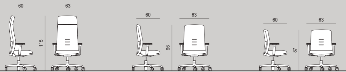
SEDUTA DIREZIONALE, SEMIDIREZIONALE E OPERATIVA IMBOTTITA | PADDED EXECUTIVE, MANAGER AND TASK ARMCHAIR
