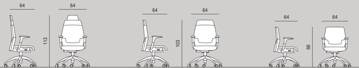
SEDUTA PRESIDENZIALE, DIREZIONALE E SEMIDIREZIONALE | PRESIDENTIAL, EXECUTIVE AND MANAGER ARMCHAIR
