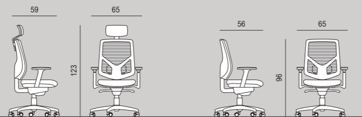
SEDUTA DIREZIONALE E OPERATIVA IN RETE | EXECUTIVE AND TASK ARMCHAIR, MESH BACKREST
