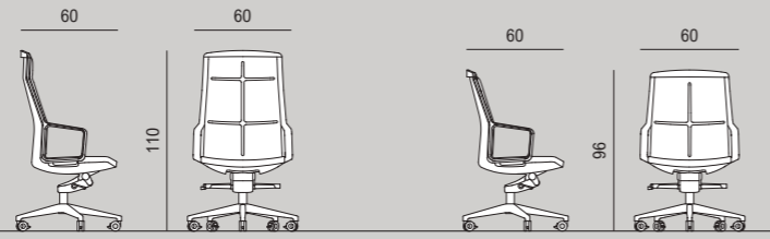
SEDUTA DIREZIONALE E SEMIDIREZIONALE IMBOTTITA | PADDED EXECUTIVE AND MANAGER ARMCHAIR
